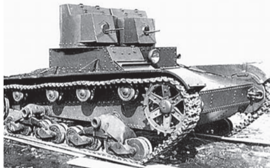
Телетанк ТТ-18 мог выполнять 16 радиоконанд.
