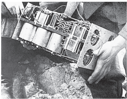
Блок управления радиоуправляемой мины «Беми».
