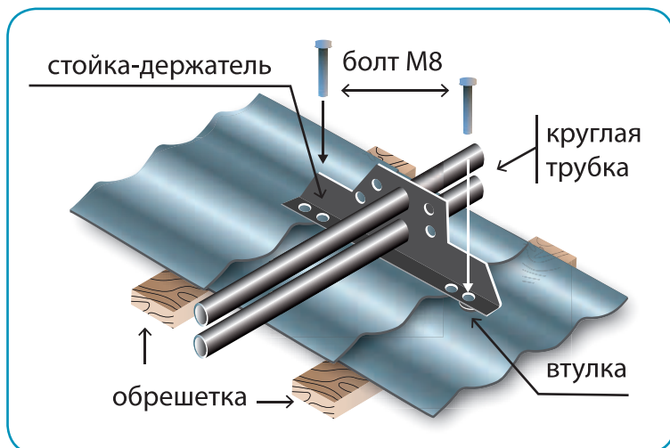
Шаг обрешетки – 30 см, как и у волны металлочерепицы. Соответственно, «мысок» (начало стойки) крепится на верхний брус, а «пятка» (конец) – на нижний.
