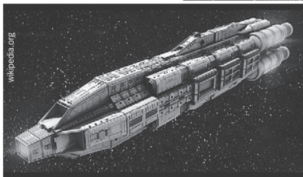
Вверху: примерно так, по расчетам, выглядит астероид. Внизу: Оумуамуа вполне может быть и вот таким длинным космическим кораблем.
